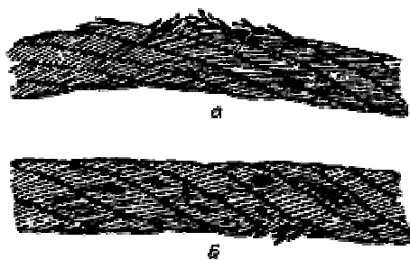
Рис. 3. Обрывы проволок в зоне уравнильного блока:
