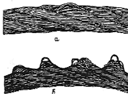
Рис. 12. Выдавливание проволок прядей:
