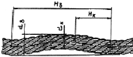
Рис. 9. Волнистость каната (объяснение в тексте)
