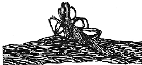
Рис. 11. Выдавливание сердечника
